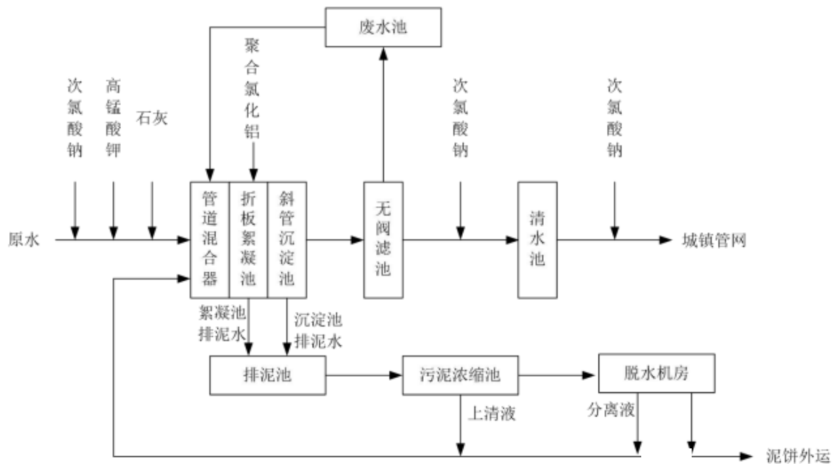
图 2-3 水厂营运期工艺流程及产污环节图
